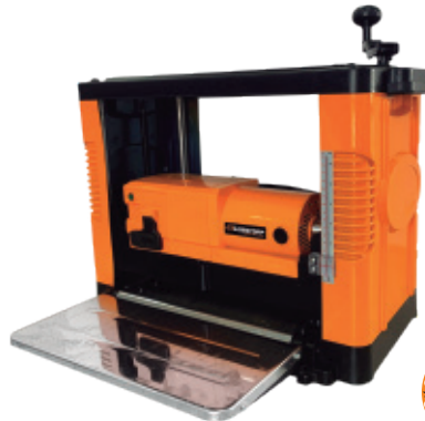
Ancho máx. de pasada 330 mm
